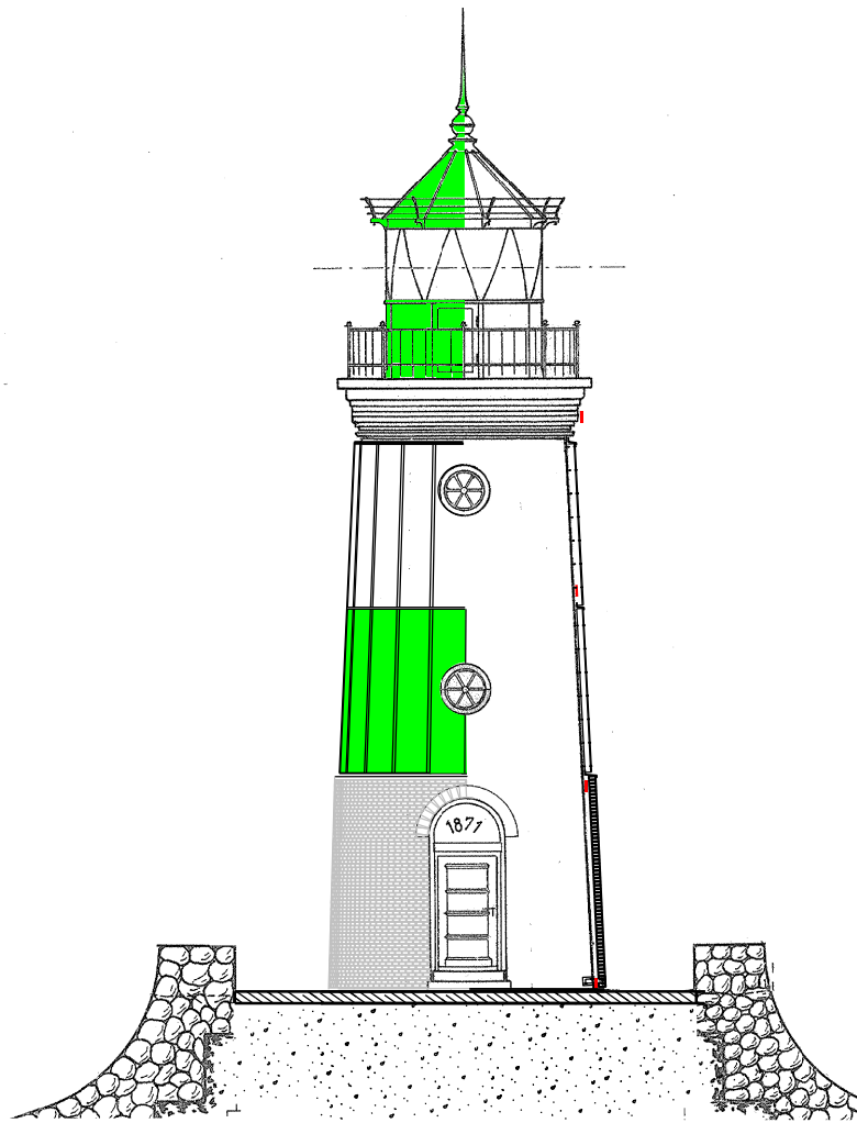
NW-Ansicht
