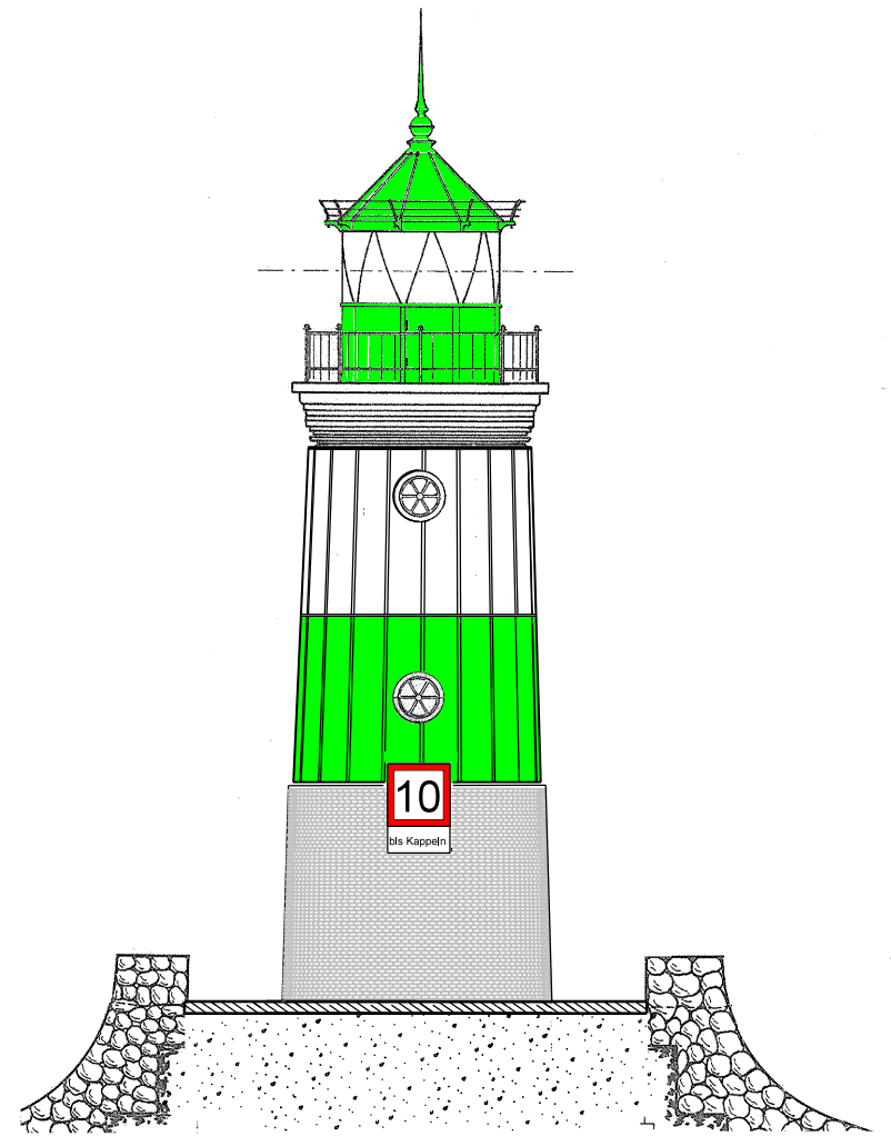
SO-Ansicht
